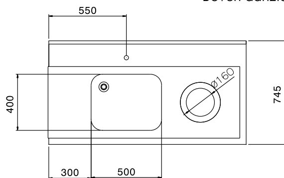
Boven aanzicht
